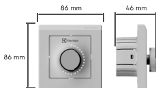
Рисунок 1. Габариты терморегулятора
