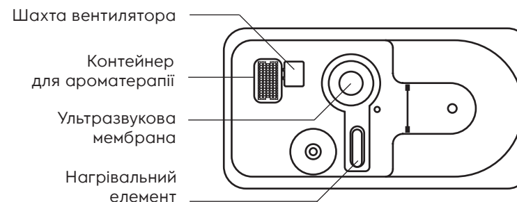
Мал. 2а Будова бази приладу
