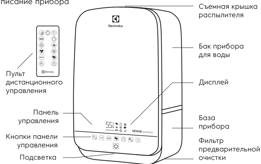
Рис. 1 Описание прибора
