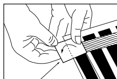
Битумная изоляция Плёнка
