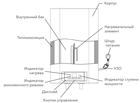
Рис. 2. Formax DL
